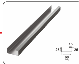
GERINC TARTÓELEM
