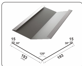
RETRO VÁPALEMENT
