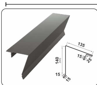
RETRO FÉLNYEREG GERINC
