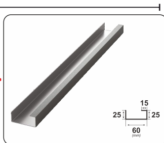
GERINC TARTÓELEM
