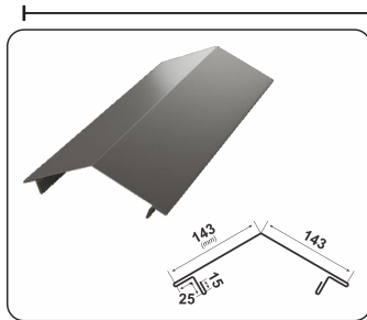
RETRO SZÖGLETES TARÉJGERINC
