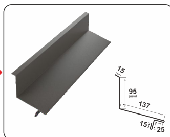
RETRO FÜGGŐLEGES FAL SZEGÉLYLEMEZ
