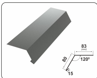
ERESZ-SZEGÉLYLEMEZ
