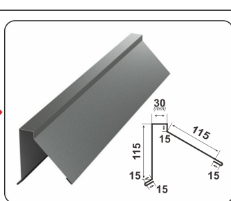
SZÖGLETES FÉLNYEREG GERINC
