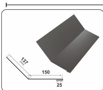
KONKÁV LEJTŐ TÖRÉSE
