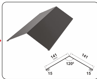
SZÖGLETES TARÉJGERINC
