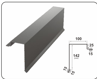
RETRO OROMDESZKA-SZEGÉLYLEMEZ
