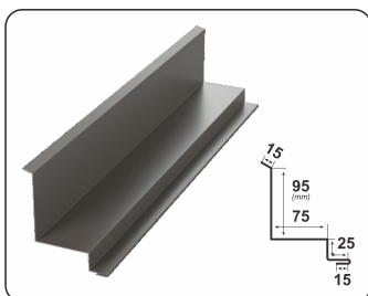
RETRO OLDALFAL SZEGÉLYLEMEZ
